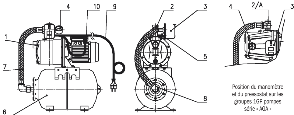
FIG. 6 Groupe 1 GP standard
