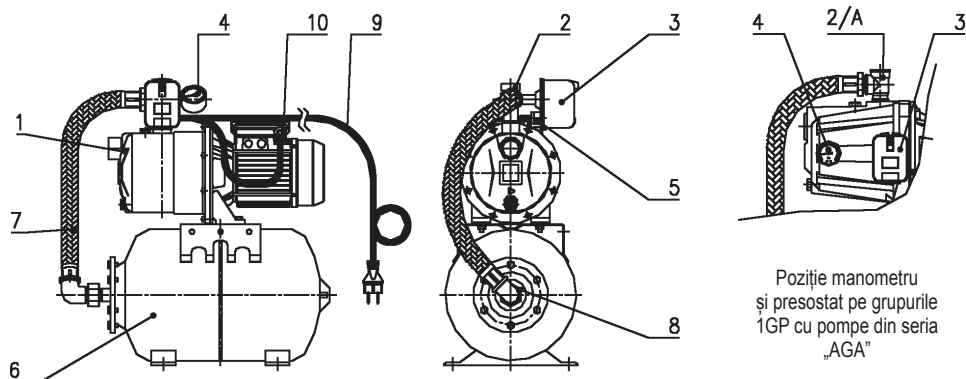
FIG. 6 Grup 1 GP standard
