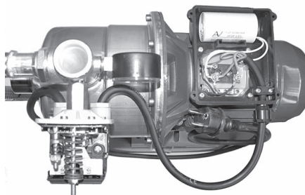
ABB. 5 Anschluss Pumpe mit Druckwächter
