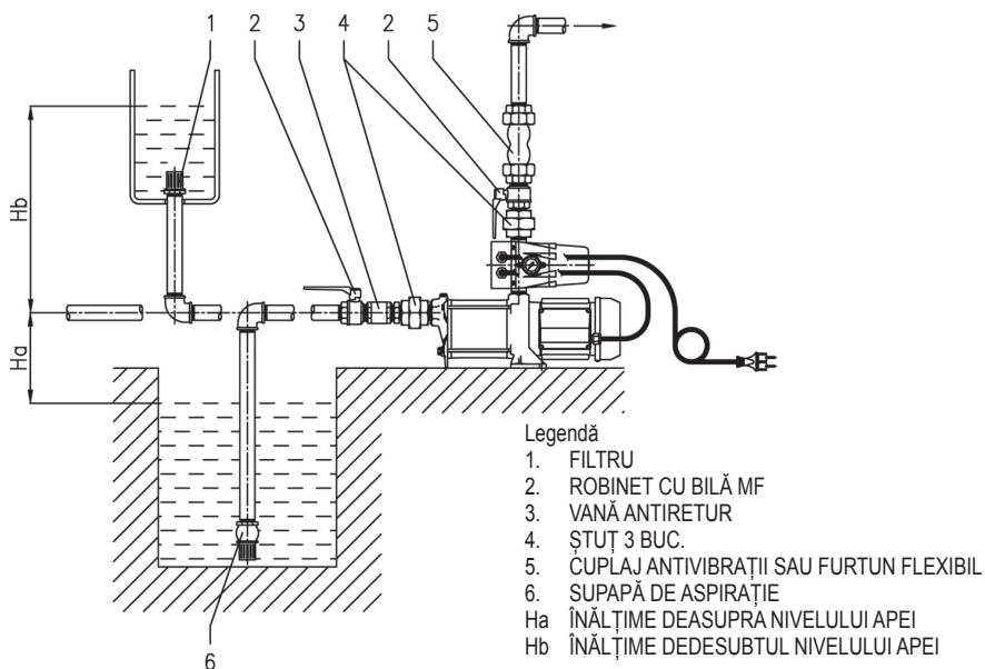
FIG. 9 Schemă tipică de instalare 1GP cu debitmetru electronic
