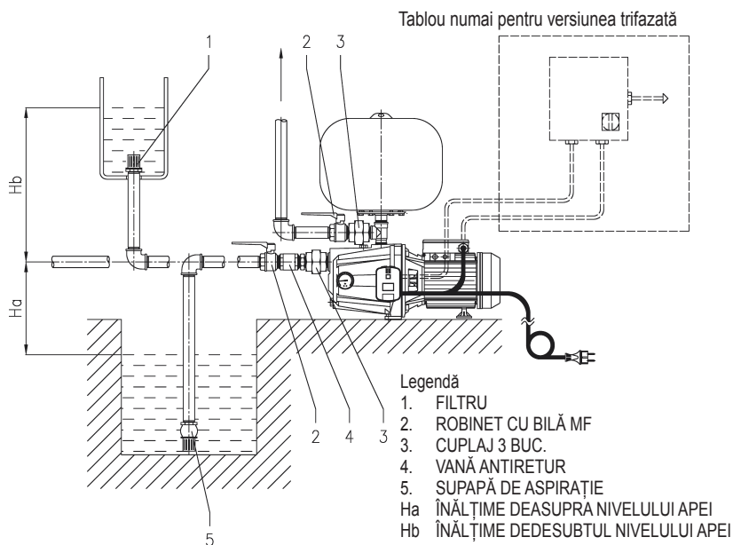
FIG. 8 Schemă tipică de instalare a grupului 1GP standard
