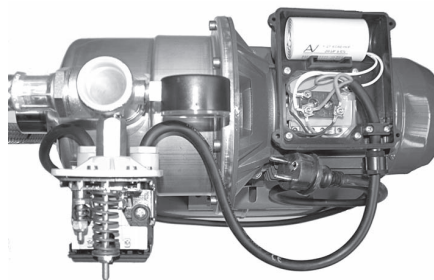
FIG. 5 Conectarea pompei cu presostat
