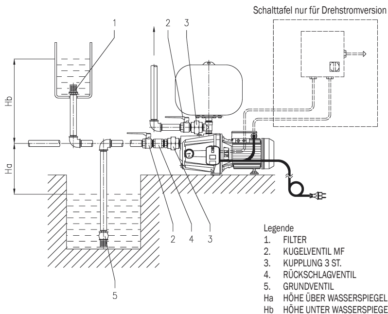
ABB. 9 Typisches Installationsschema 1GP mit elektronischem Flusswächter
